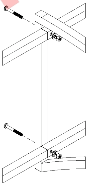
E (1:5)
