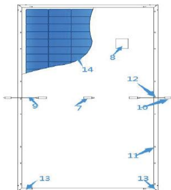
Фигура 1 Разрез на модула - Конструкция и компоненти
